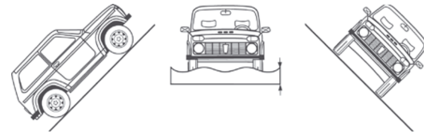
58% Steigfähigkeit
